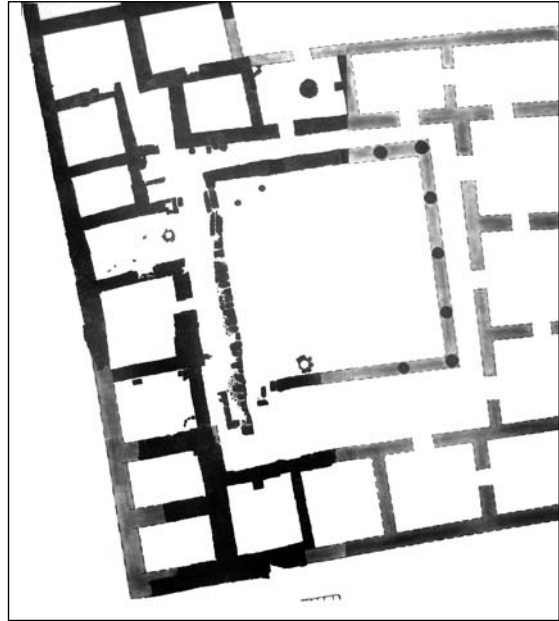
איור 2. תכנית המבנה מן התקופה הרומית
